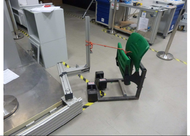
Res.8/Pic.8: Arkadan Öne Yatay Dayanıklılık Testi Back Forward Horizontal Durability Test
